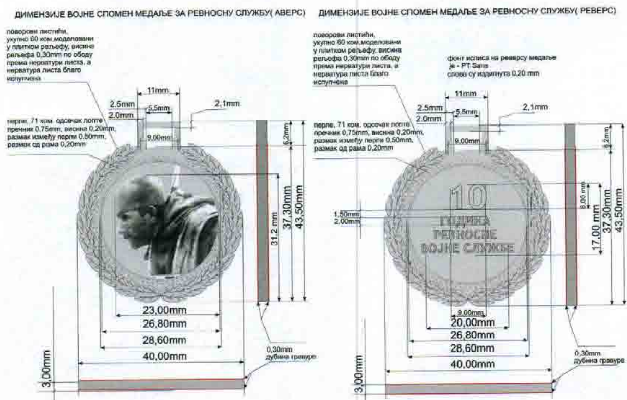
Слика 3. Димензије аверса и реверса војне спомен-медаље за ревносну службу - 10 година
